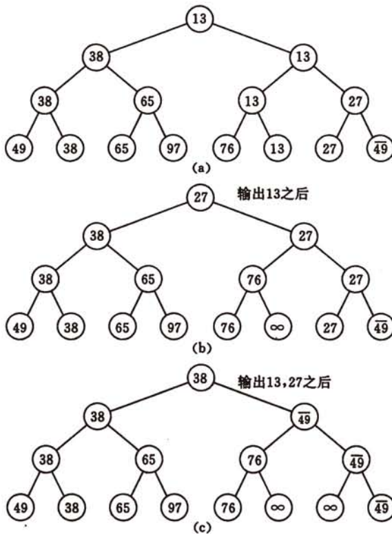
图 10.9 树形选择排序示例
