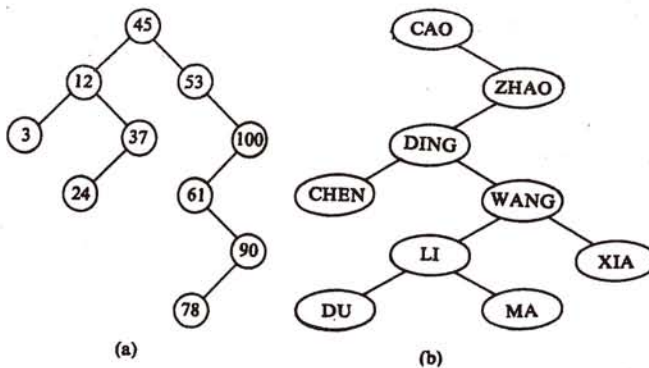
图 9.7 二叉排序树示例
