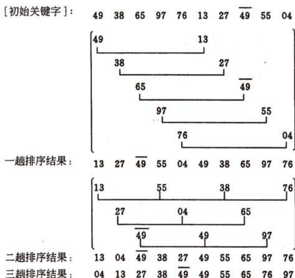
图 10.5 希尔排序示例
