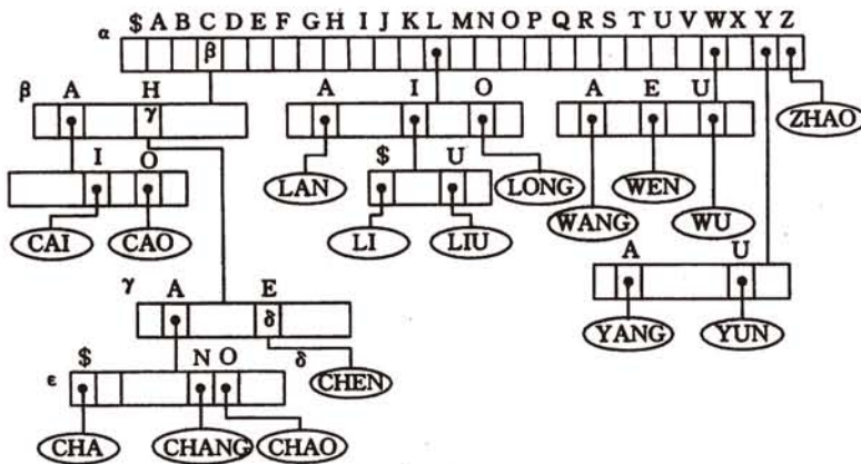
图 9.21 表示(9-24)关键字集的 Trie 树(深度=5)
