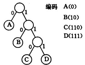
图 6.25 前缀编码示例
