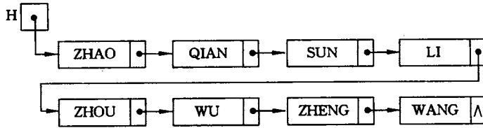
图 2.6 线性链表的逻辑状态
