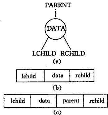
图 6.7 二叉树的结点及其存储结构 (a) 二叉树的结点; (b) 含有两个指针域的结点结构; (c) 含有三个指针域的结点结构
