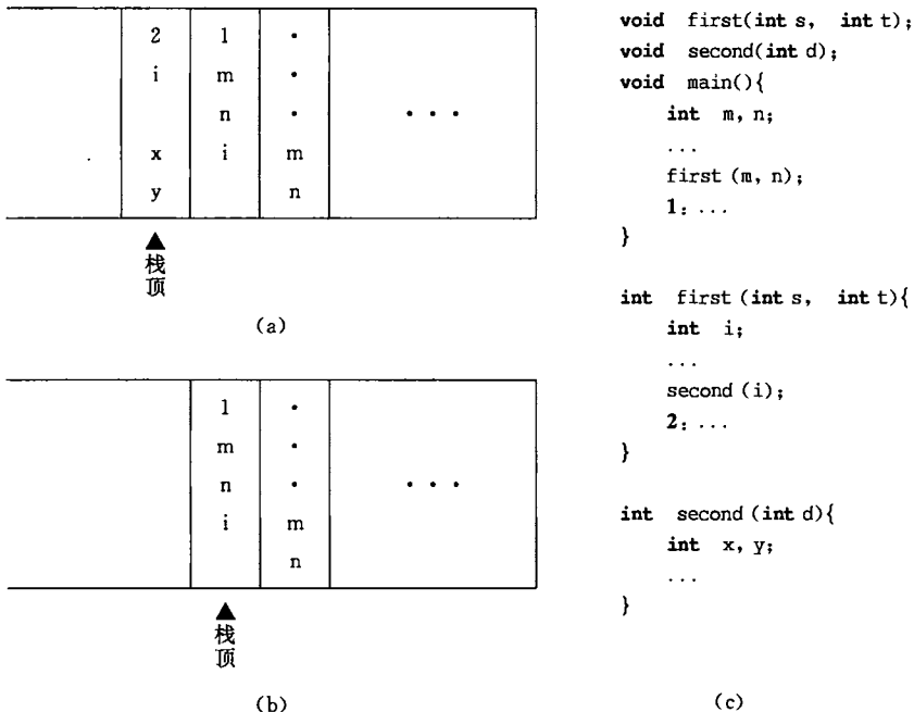
图 3.6 主函数 main 执行期间运行栈的状态
