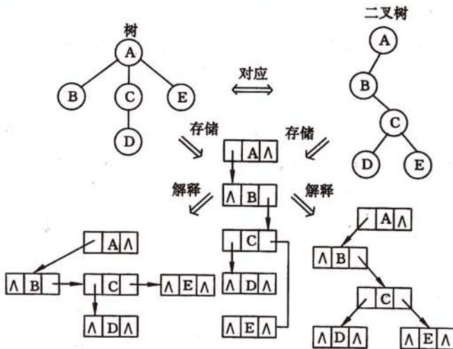
图 6.16 树与二叉树的对应关系示例
