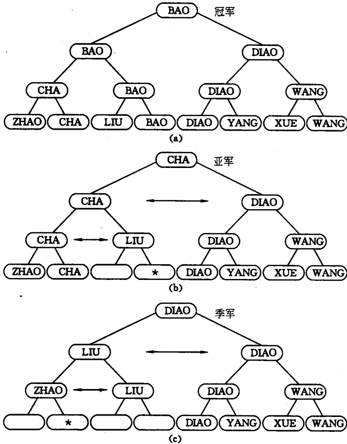
图 10.8 锦标赛过程示意图 (a) 选拔冠军的比赛程序; (b) 选拔亚军的两场比赛; (c) 选拔季军的两场比赛
