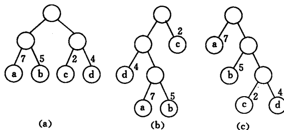
图 6.22 具有不同带权路径长度的二叉树
