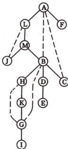
图 7.20 G_5 的深度优先生成树
