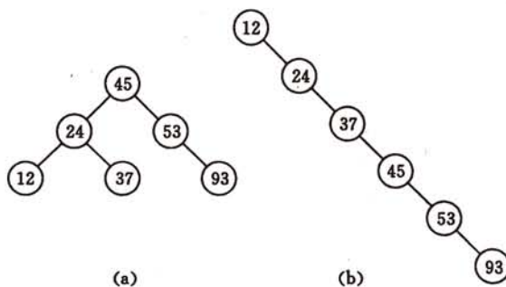
图 9.10 不同形态的二叉查找树
