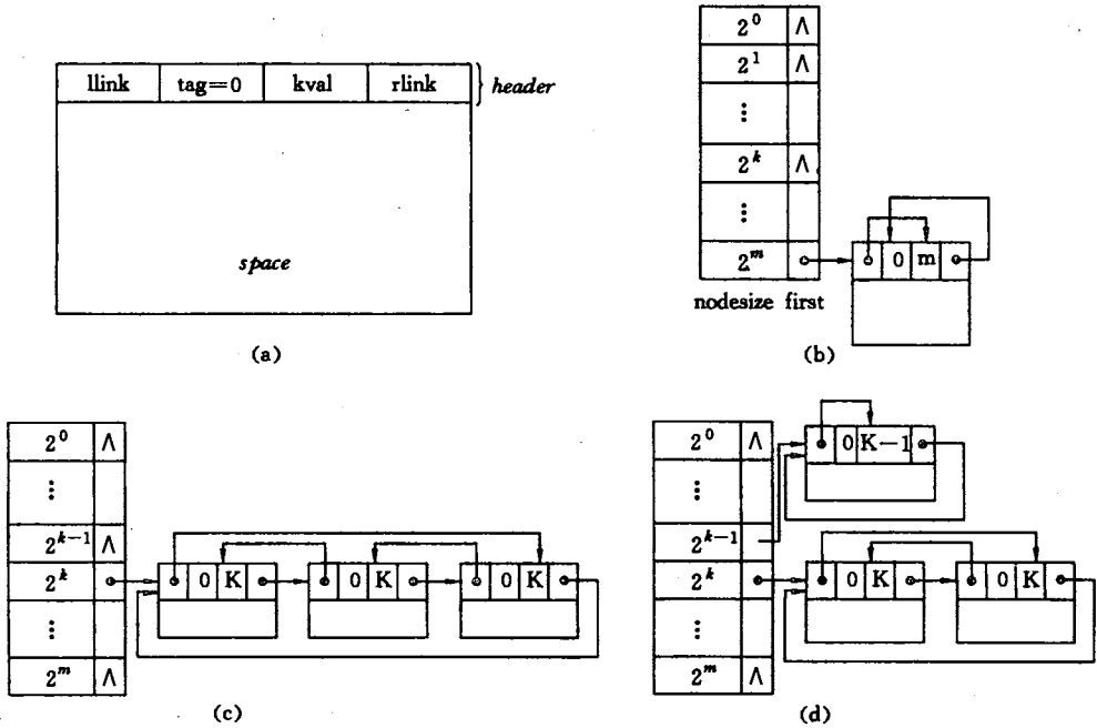
图 8.8 伙伴系统中的可利用空间表 (a) 空闲块的结点结构; (b) 表的初始状态; (c) 分配前的表; (d) 分配后的表
