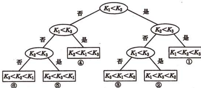
图 10.16 描述排序过程的判定树
