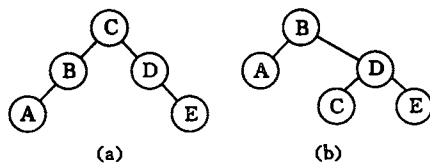
图 9.5 根的权小于子树根权的情况
