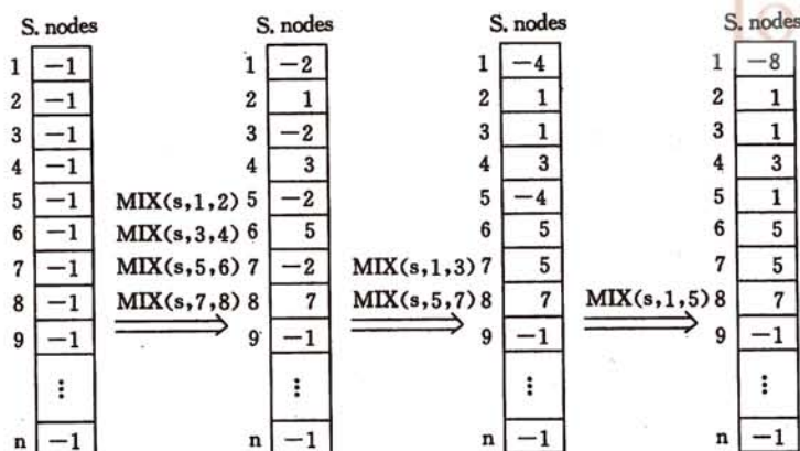
图 6.20 求等价类过程示例
