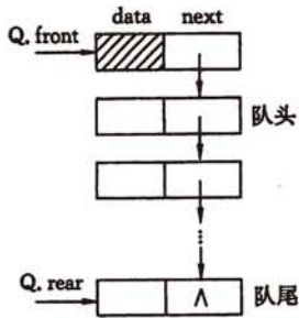
图 3.10 链队列示意图
