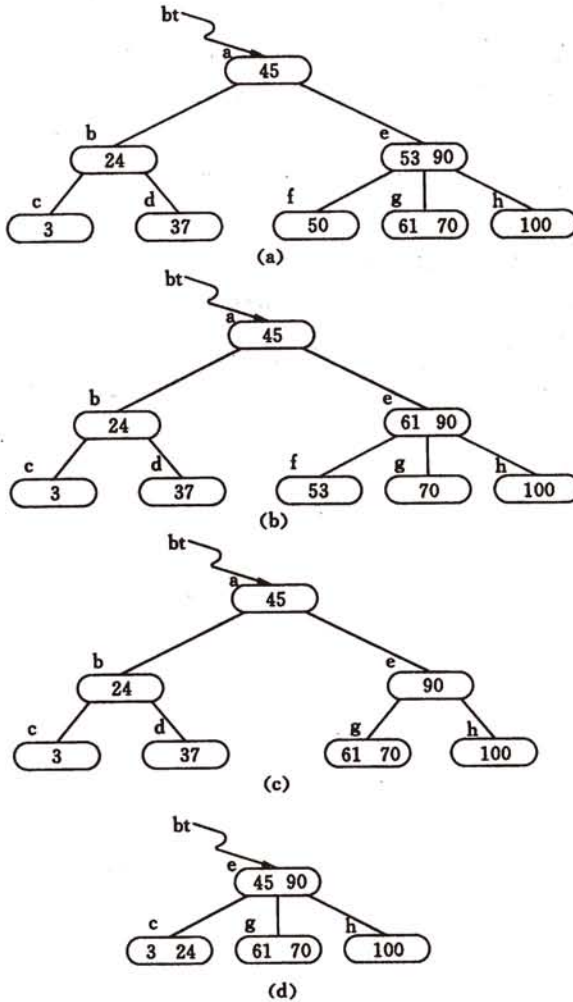
图 9.17 在 B-树中删除关键字的情形
