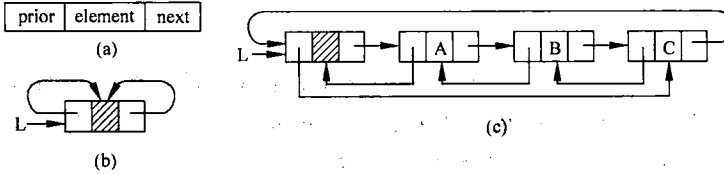
图 2.14 双向链表示例
