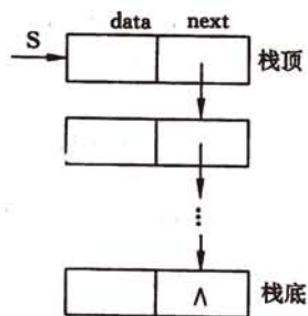
图 3.3 链栈示意图
