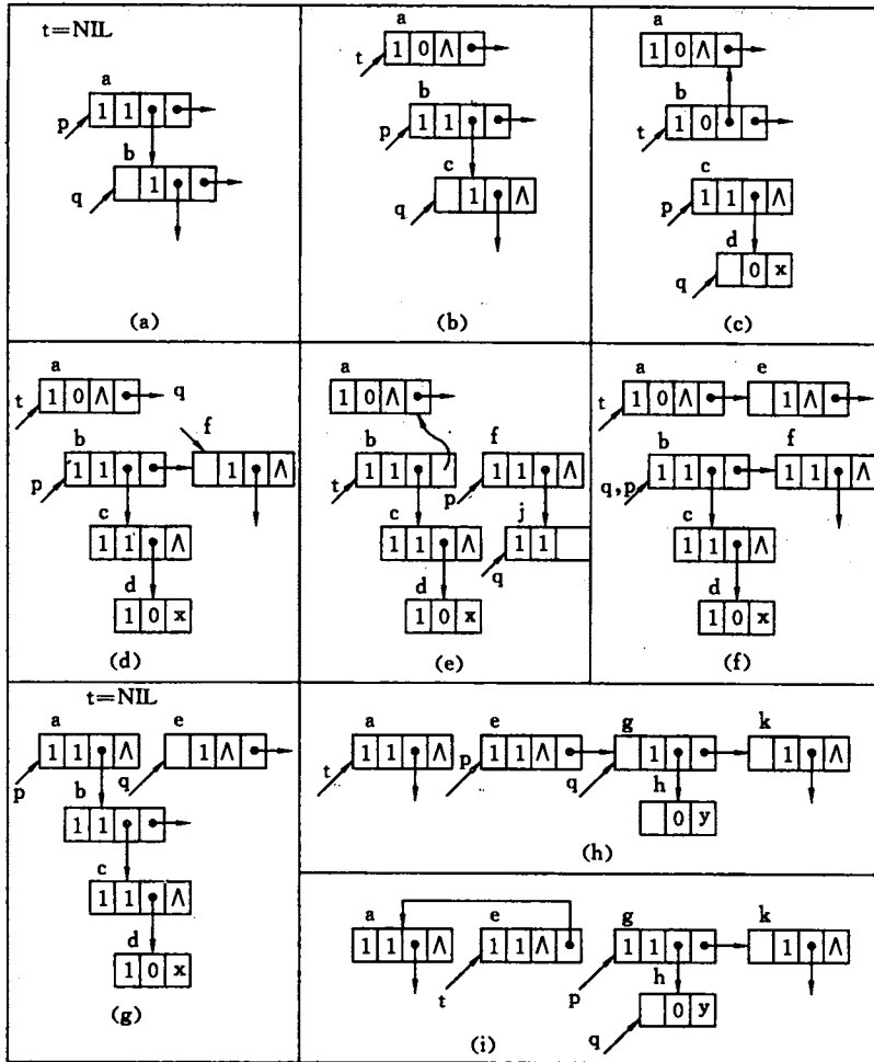
图 8.11 遍历广义表
