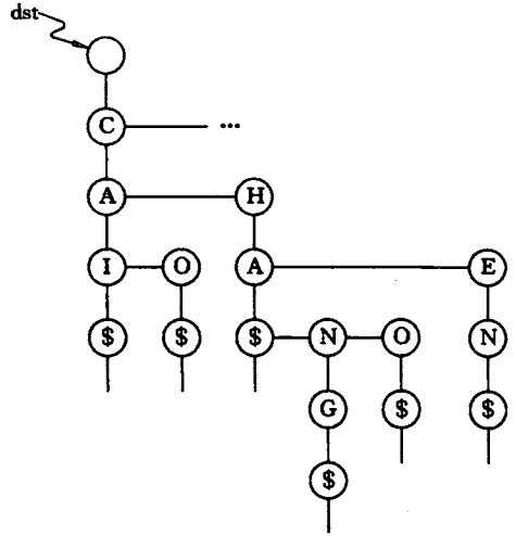
图 9.20 双链树示例
