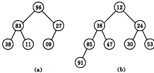
图 10.10 堆的示例
