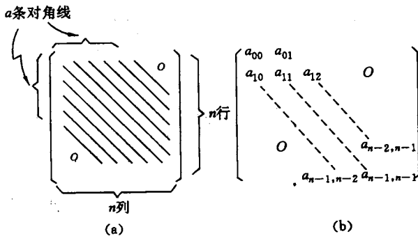
图 5.4 对角矩阵
