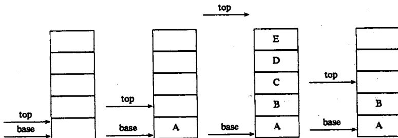
图 3.2 栈顶指针和栈中元素之间的关系
