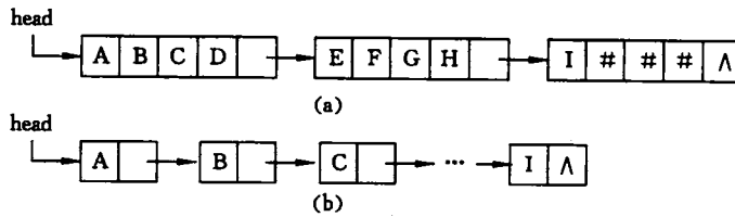
图 4.2 串值的链表存储方式
