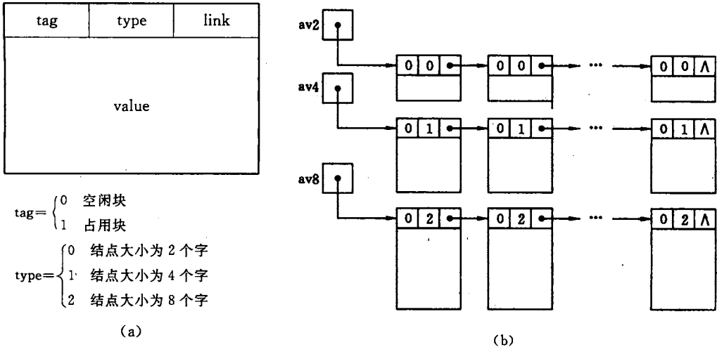
图 8.3 有 3 种大小结点的可利用空间表 (a) 结点结构; (b) 可利用空间表
