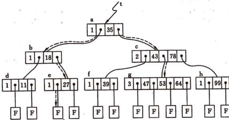
图 9.14 一棵 4 阶的 B-树
