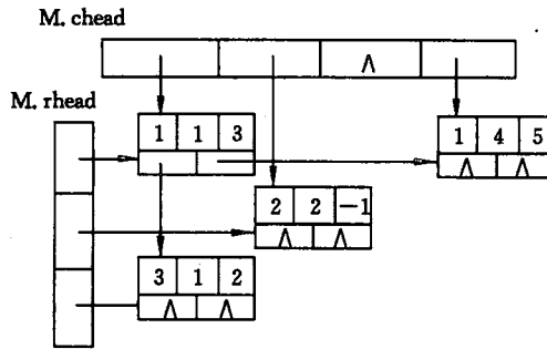
图 5.6 稀疏矩阵 M 的十字链表
