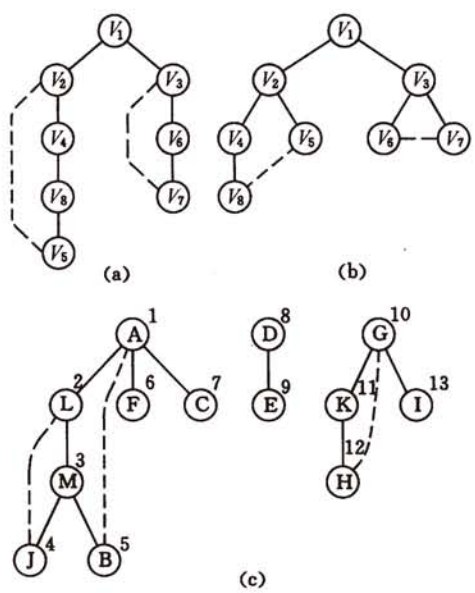
图 7.15 生成树和生成森林
