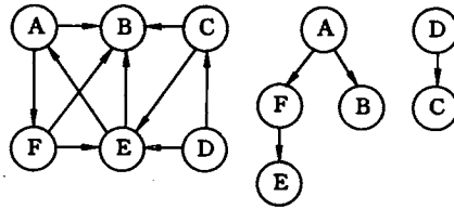
图 7.6 一个有向图及其生成森林
