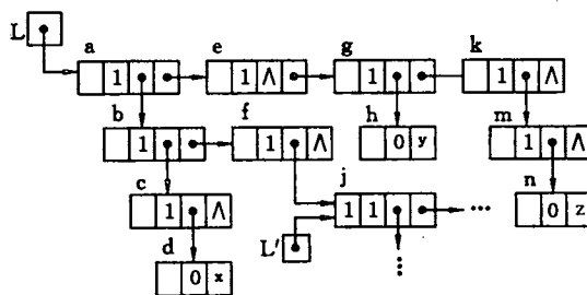
图 8.10 待遍历的广义表
