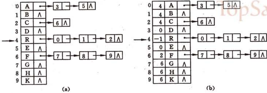
图 6.14 图 6.13 的树的另外两种表示法 (a) 孩子链表; (b) 带双亲的孩子链表
