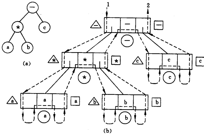
图 6.10 3 种遍历过程示意图 (a) 表达式 (a * b - c) 的二叉树; (b) 遍历的递归执行过程
