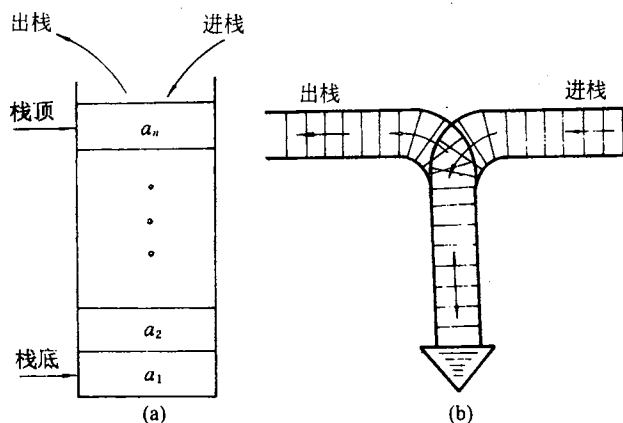
图 3.1 栈
