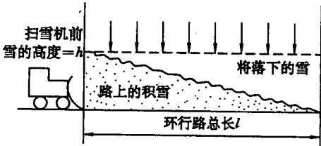
图 11.7 环形路上扫雪机系统平衡时的状态
