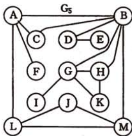
图 7.19 连通图 G_5
