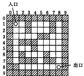
图 3.4 迷宫
