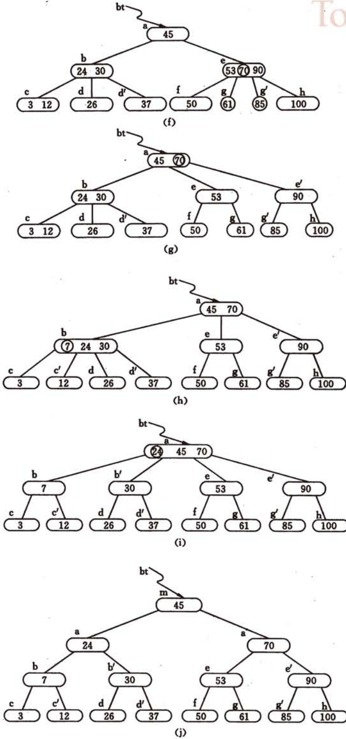
图 9.16 (续)
