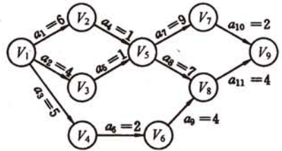
图 7.29 一个 AOE-网
