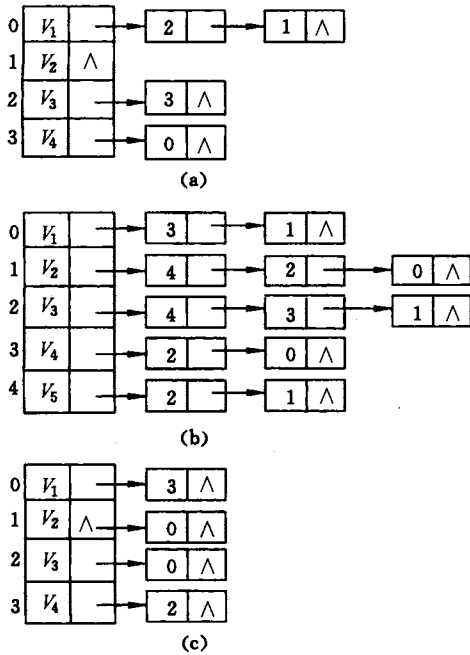
图 7.10 邻接表和逆邻接表 (a) G_1 的邻接表; (b) G_2 的邻接表; (c) G_1 的逆邻接表
